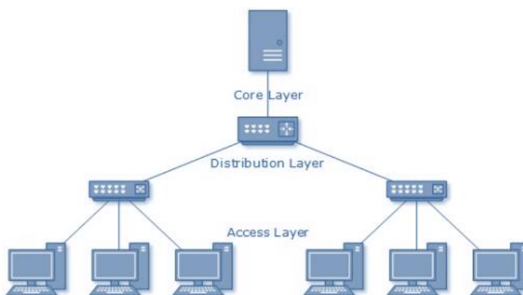
Gambar 1. 7 Topologi Pohon
