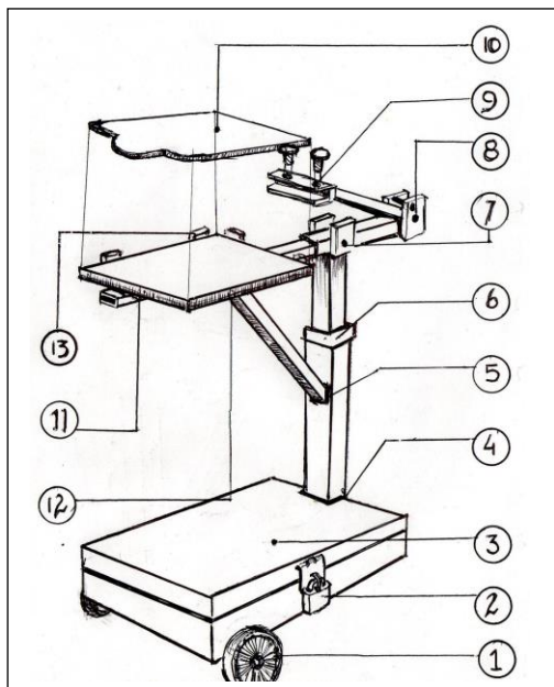
Gambar 4. Gambar Perspektif
