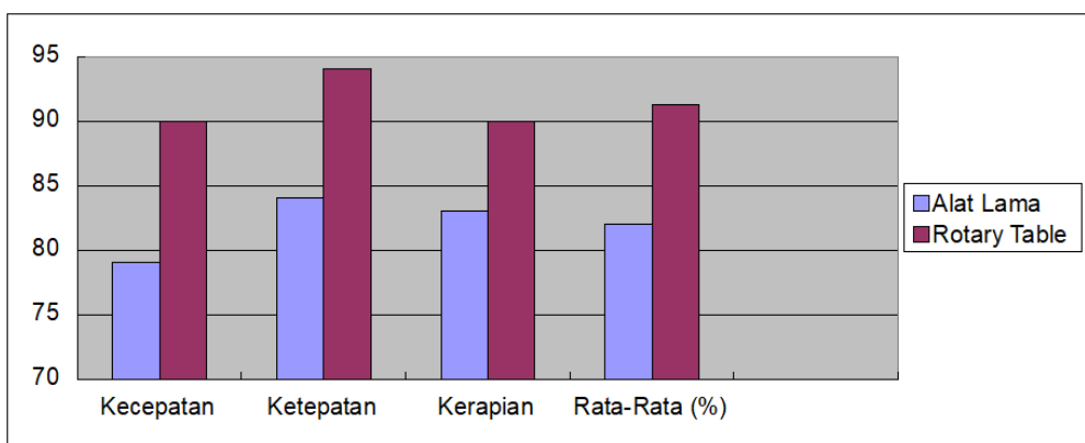
Gambar 6. Grafik Perbandingan Keefektifan Antara Alat Lama dengan Alat Rotary Table
