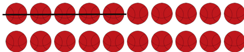
Gambar.2.1.3.4. Himpunan bola
