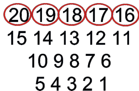
Gambar.2.1.3.3 garis bilangan
