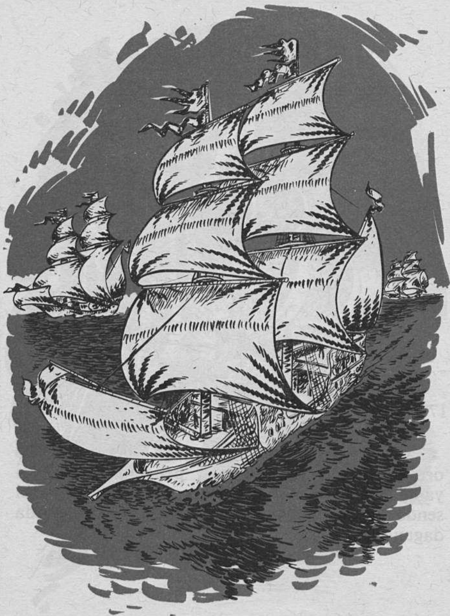
Kapal-kapal perang Portugis berlayar ke Laut Merah.
