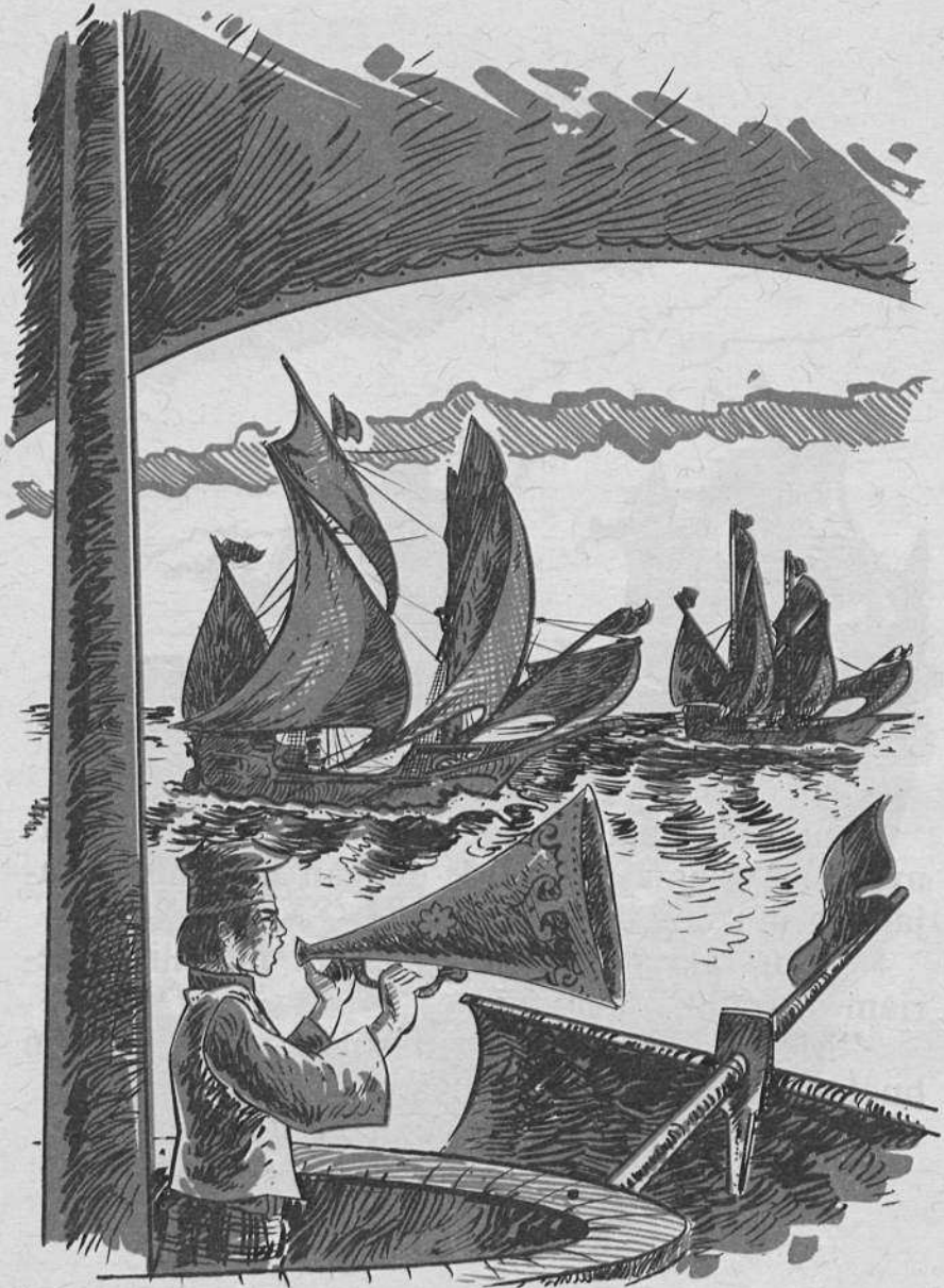
Suara azan berkumandang dari setiap kapal Aceh.
