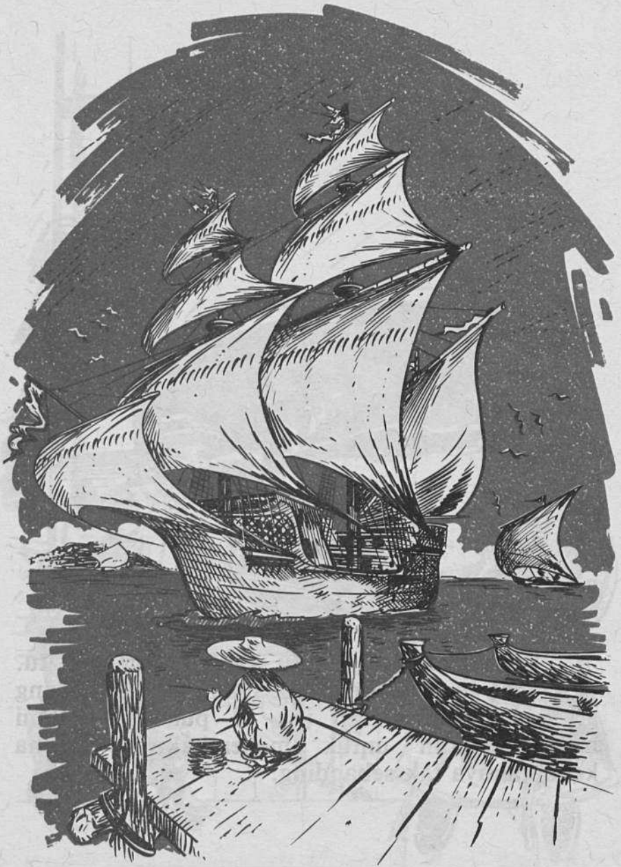
Kapal Portugis itu kembali ke pangkalannya di bandar Malaka.
