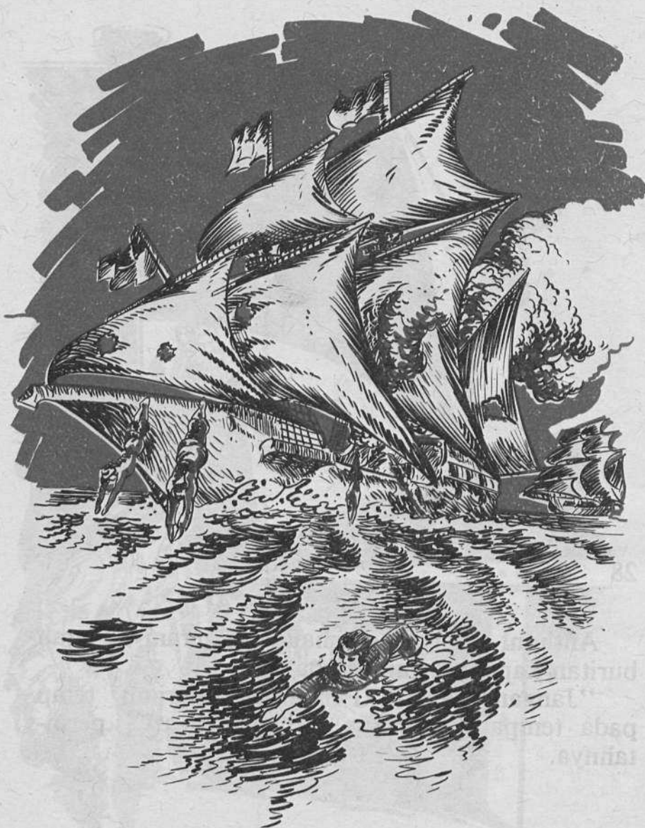
Sebuah kapal Aceh terbakar dan tenggelam.
