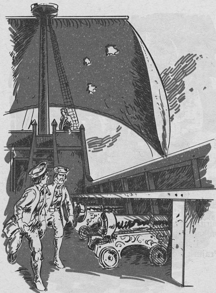
Anthoni Galavalo memandang geram ke arah buritan kapalnya yang terbakar.
