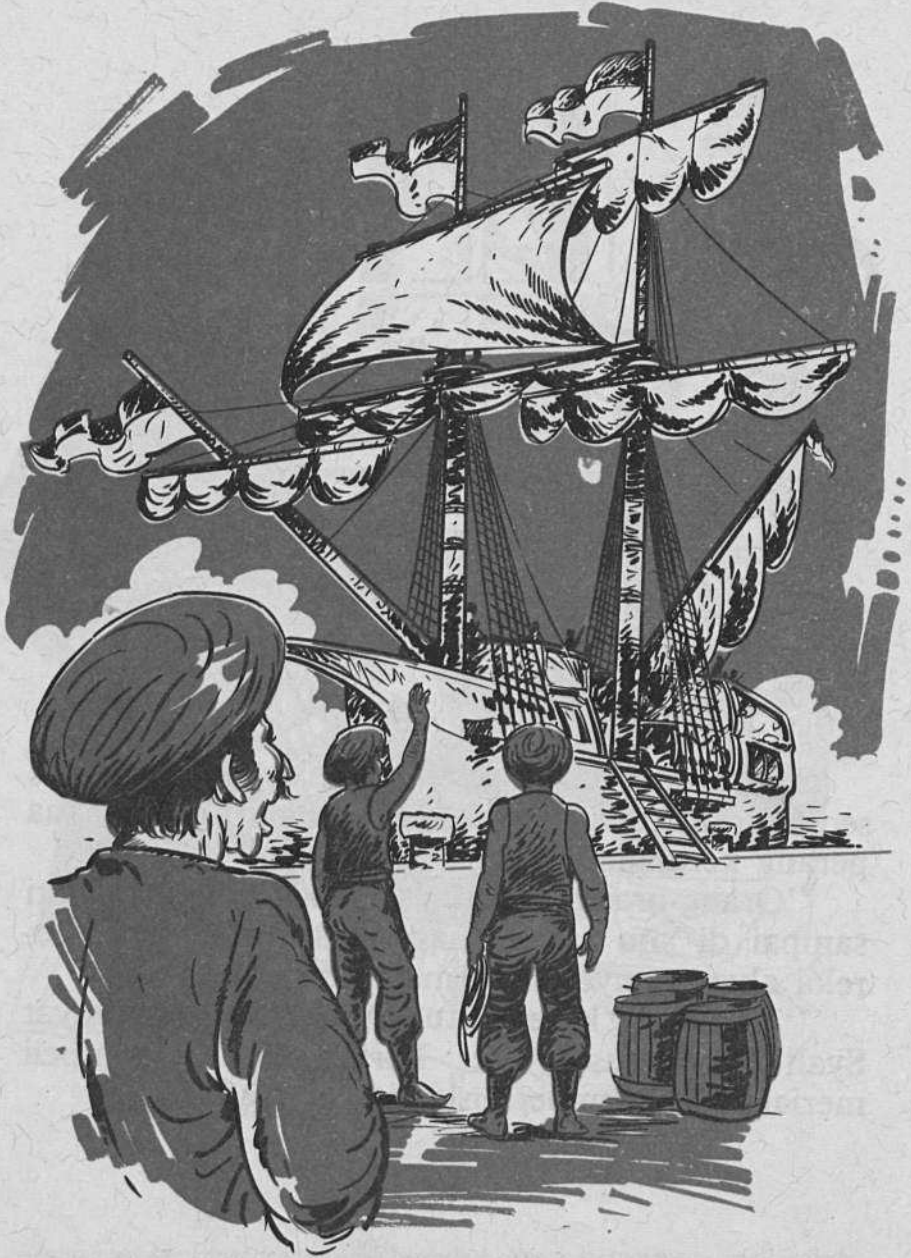
Armada dagang Aceh mendarat di bandar Turki.
