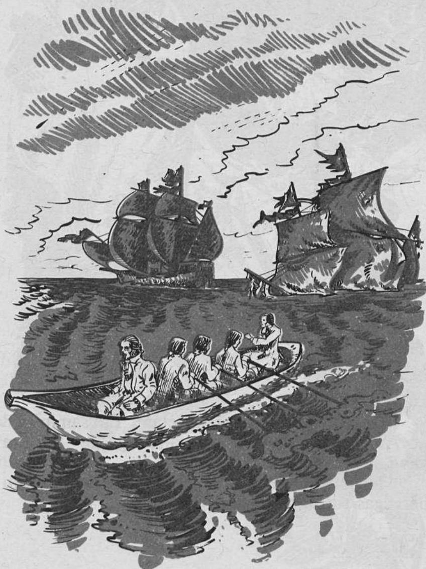
Anthoni Galavalo dengan lima orang stafnya menyelamatkan diri dengan perahu.
