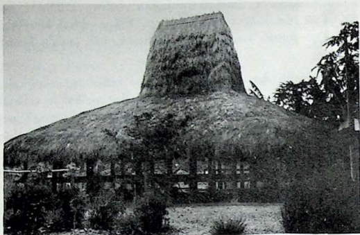
Contoh rumah adat (belum diberi dinding) yang sudah mempergunakan fondasi beton. Rumah adat itu didirikan di Parai Liu yang terletak di pinggiran kota Waingapu, Sumba Timur.
