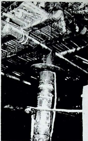
Bagian-bagian tiang utama (soko guru) rumah adat gaya Sumba Timur.
