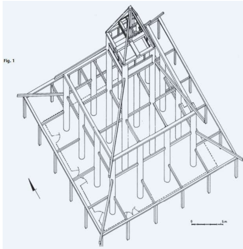
Gambar 8.3 Sketsa Masjid Agung Demak 39 Sumber: Njoto, 2015
