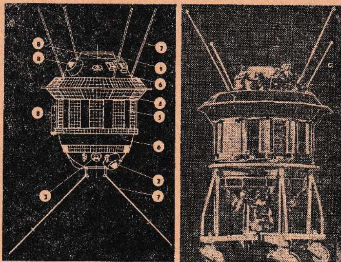
Foto dari stasiun antarplanet otomatis diatas trolis-pemasangannya dan diagram stasiun ini : (1) tingkap kamera, (2) motor sistim orientasi, (3) monitor matahari, (4) seksi baterai matahari, (5) sisim penguntji kontrol-panas, (6) layar 2 pelindung panas, (7) antena, (8) pesawat 2 research.
