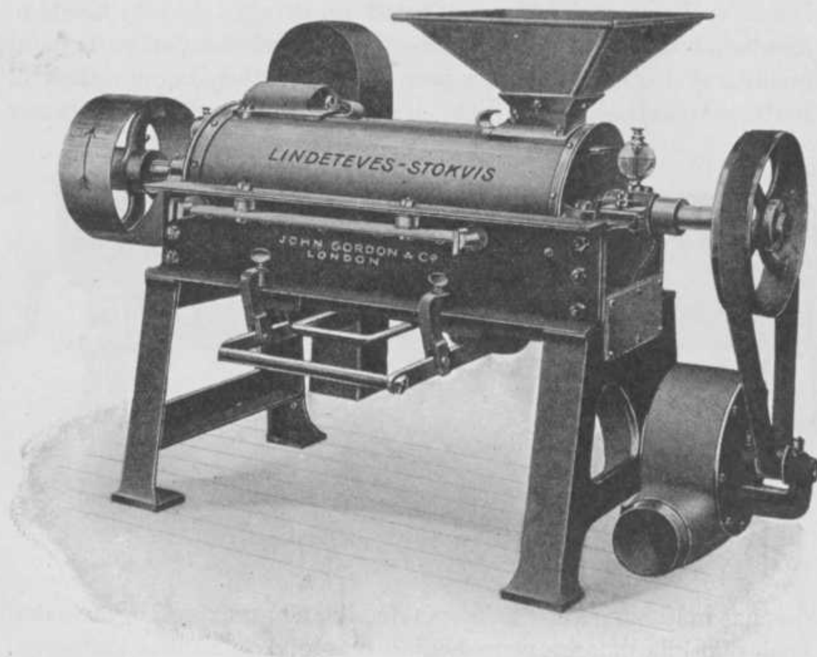
Gamb. 22. Mesin pembelah.
