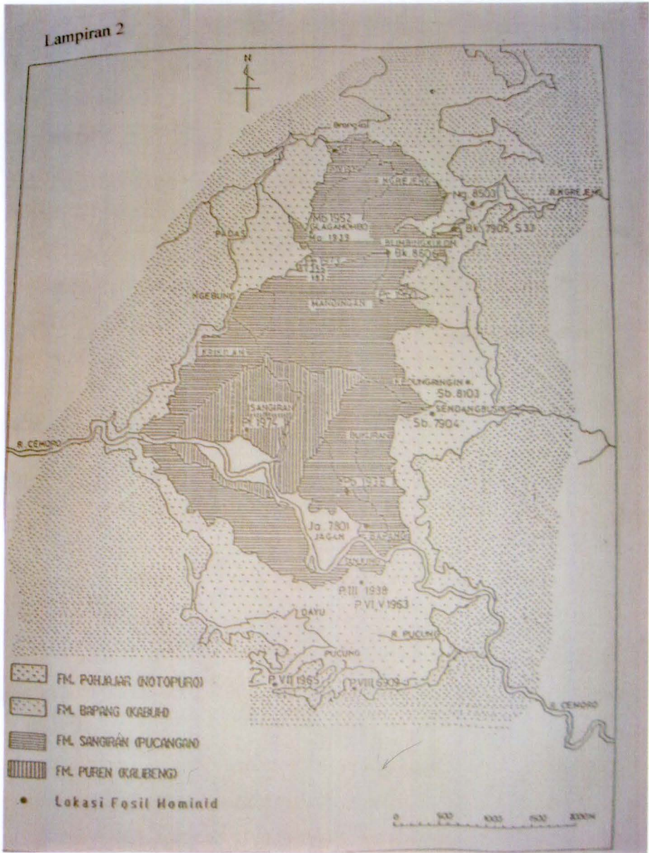
Peta Geologi Daerah Sangiran Repro dari Azizet al, 1994
